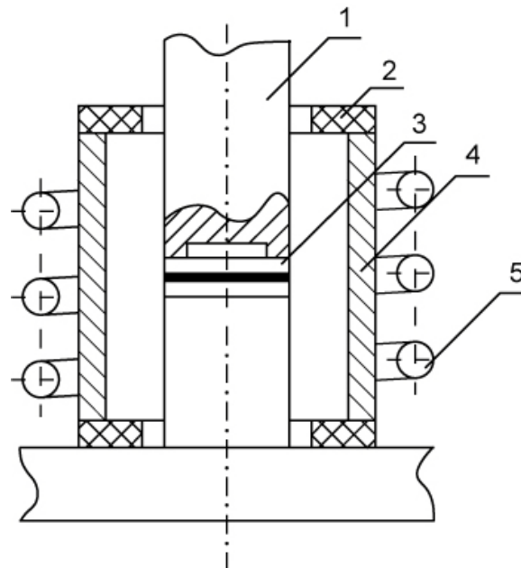
Фиг.4 Системата за индиректно радиационно нагряване: 1 – Притискач; 2 – Изолатор; 3 - Заварявано съединение; 4 – Гръбен детайл; 5 Индуктор
